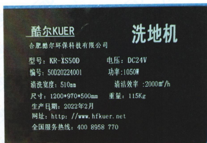
洗地机铭牌
