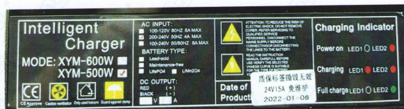
充电器铭牌
